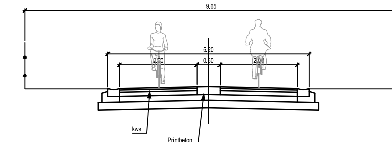
TYPEDWARSPROFIEL 23
